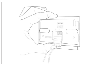
Fig. 3 Fixați temporar REMOCON NET MINI pe placă folosind cărțile dedicate.
