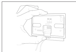
Afb. 3 De REMOCON NET MINI voorlopig op de plaat bevestigen met behulp van de daartoe voorziene haken.
