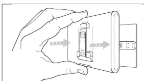
Abb. 5 Nehmen Sie das REMOCON NET MINI aus der provisorischen Position (Abb. 2) und befestigen Sie das Gateway an der Platte, indem Sie auf die Seiten drücken, bis das Einrasten der vier gleichen Seitenhaken nicht mehr zu spüren ist.
