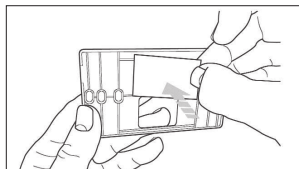
Fig. 1b Applicare il bi-adesivo dietro la piastrina di supporto, rimuoverne la patina protettiva e fissarlo sulla lamiera della caldaia;
