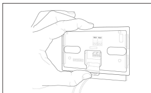
Fig. 3 Fixer temporairement le REMOCON NET MINI à la plaque au moyen des crochets prévus à cet effet.
