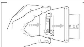
Fig. 5 Scoateți REMOCON NET MINI din poziția sa temporară (fig.2) și fixați-l pe placă, aplicând presiune pe părțile laterale până când cele patru cârlige laterale mici se fixează.
