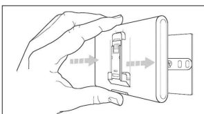
Fig. 5 Fjern REMOCON NET MINI fra den midlertidige placering (fig. 2), og gør den fast til pladen ved at trykke langs de to sider, indtil de fire små sidekroge udsender et klik.
