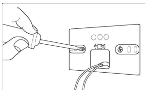
Fig. 1 Fixați placa de susținere pe perete cu ajutorul șuruburilor furnizate
