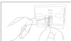
Fig. 4 Forbind ledningsparret fra konnektoren på BUS BridgeNet-kortet på fyret til BUS BridgeNet på REMOCON NET MINI-konnektoren (overhold polariteten B med B og T med T)*. * plastikfanen kan fjernes for at lette tilslutningen af ledningerne, sådan som vist i figuren.
