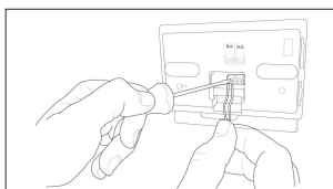
Fig. 4 Conectați perechea de cabluri de la BUS BridgeNET de pe placa de circuit a centralei la conectorul BUS BridgeNET de pe REMOCON NET MINI (respectând polaritățile B la B și T la T) *
