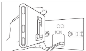
Afb. 2 De REMOCON NET MINI omdraaien.
