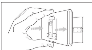
Fig. 5b Fixați-l pe placă aplicând presiune de-a lungul laturilor;
