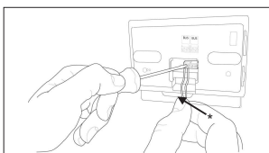
Abb. 4 Verbinden Sie das Adernpaar des Steckers BUS BridgeNET auf der Heizplatte mit dem Anschluss BUS BridgeNet des REMOCON NET MINI (unter Beachtung der Polarität B mit B und T mit T)*.
