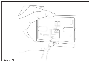
Fig. 3 Sæt samtidig REMOCON NET MINI fast på holdepladen ved hjælp af krogene.
