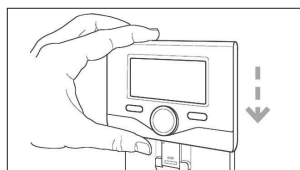
Abb. 6 (optional) Legen Sie das REMOCON PLUS auf die Basis und drücken Sie ihn vorsichtig hinunter.
