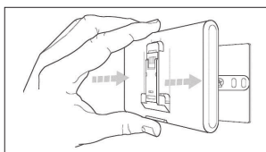
Fig. 5 Retirer le REMOCON NET MINI de sa position temporaire (fig. 2) et le fixer à la plaque en appuyant sur les côtés jusqu'au déclic indiquant l'engagement des quatre petits crochets latéraux.
