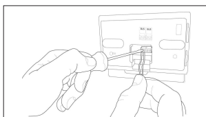
Afb. 4 Het dradenpaar van de BridgeNet BUS-connector op de ketel-kaart met de BridgeNet BUS-connector van de REMOCON NET MINI verbinden (de polariteit B met B en T met T in acht nemen)*
