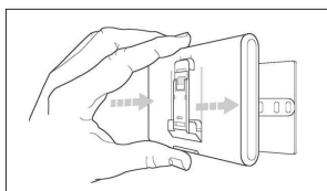
Afb. 5b Het apparaat op de steunplaat bevestigen door stevig op de zijkanalen te drukken.
