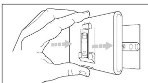
Afb. 5 De voorlopig aangebrachte REMOCON NET MINI (afb. 2) verwijderen en het apparaat op de plaat bevestigen door stevig op de zijkanalen te drukken totdat u de vier kleine haakjes aan de zijkanalen hebt horen klikken.
