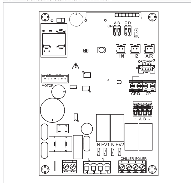
A Scheda elettronica INN-FR-B32
