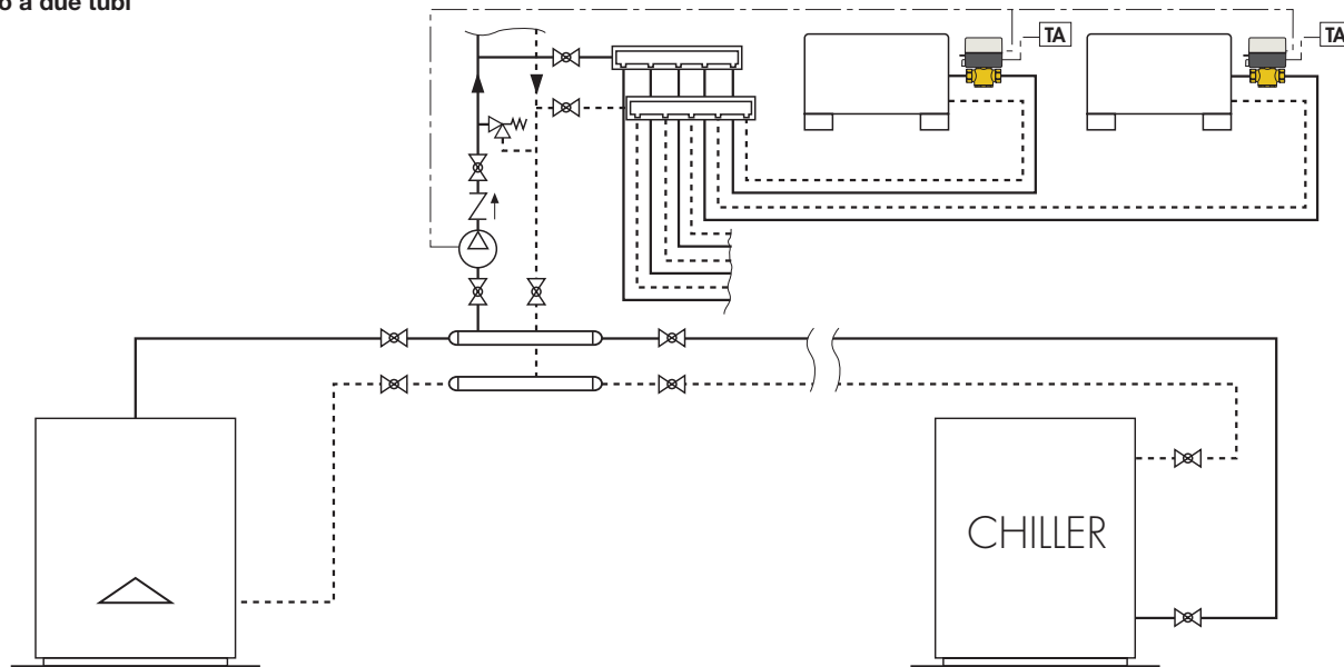
Impianto a due tubi
