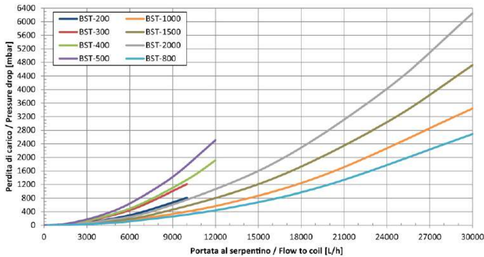
Perdite di carico sul serp. solare
