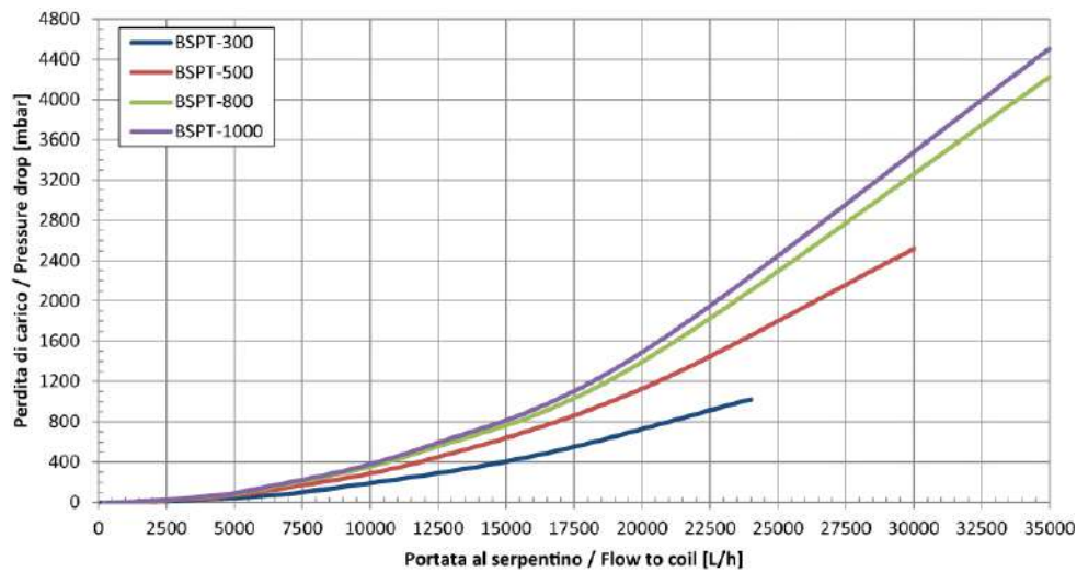
Perdite di carico sul serp.PdC
