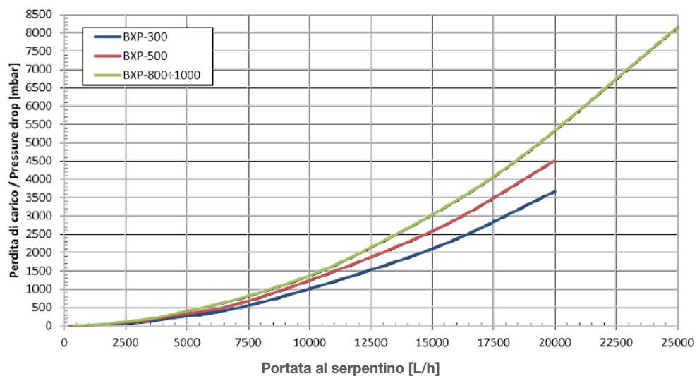
Perdita di carico al serpentino
