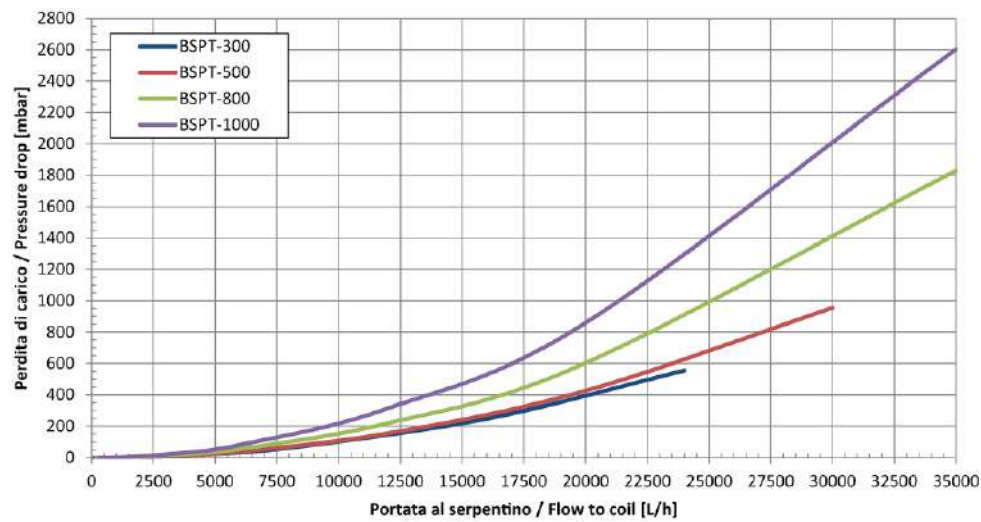
Perdite di carico sul serp. integr.
