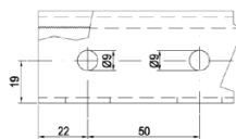
Vista laterale/Side view Vue de côté/Vista lateral
