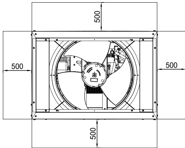
SPAZIO MINIMO NECESSARIO MANUTENZIONE MINIMUM REQUIRED MAINTENANCE
