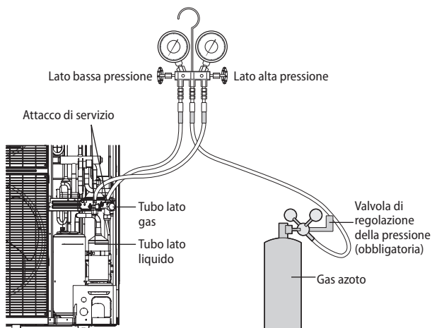
Manometro del collettore
